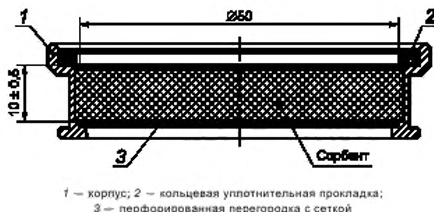
Рисунок 4 — Секция колонки с сорбентом
