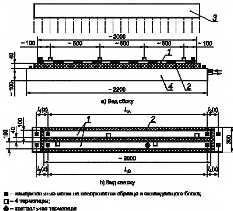
1 — образцы (А и В); 2 — теплоизоляция (пеностекло); 3 — источник инфракрасного излучения; 4 — металлический блок с охлаждающей водой
