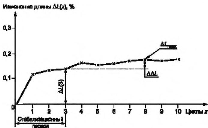
Рисунок 2 — Пример определения формоустойчивости образца
