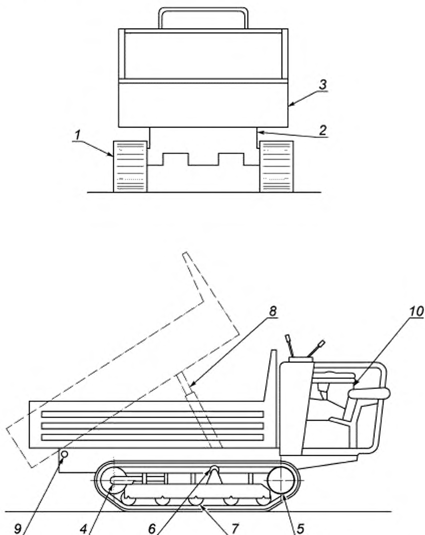
1 — гусеница; 2 — основная рама; 3 — кузов; 4 — ленивец; 5 — приводная звездочка; 6 — поддерживающий ролик; 7 — ролик гусеницы; 8 — гидроцилиндр разгрузки; 9 — ось шарнира кузова; 10 — энергетическая установка
