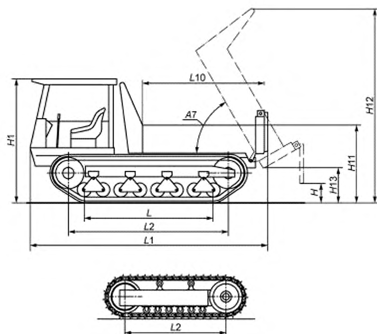
Рисунок 30 (лист 2)
