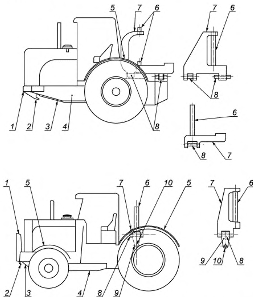
1 — бампер, 2 — тяговый крюк, 3 — защита днища; 4 — основная рама; 5 — крыло; 6 — поворотный шкворень; 7 — крепёжная вилка; 8 — ось шарнира, 9 — хомут, крепёж; 10 — оси переднего и заднего шарниров
