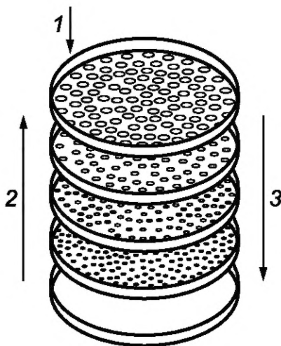
1 — загрузка испытываемого материала; 2 — направление увеличения диаметра отверстий; 3 — направление движения материала
