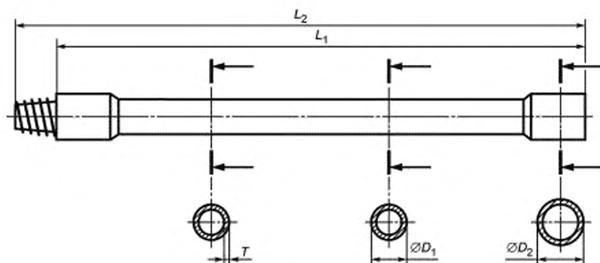
Рисунок 5 — Бурильная труба
