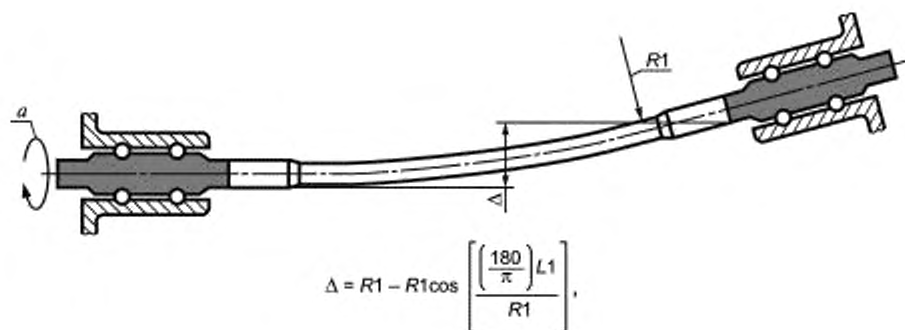
R1 — испытательный радиус, α — вращение
