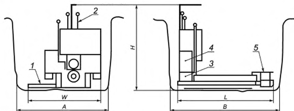
A — ширина колодца; B — длина колодца; H — общая высота машины; L — общая длина машины; W — общая ширина машины; 1 — место оператора; 2 — управление процессом бурения; 3 — шпиндель; 4 — каретка; 5 — зажим
