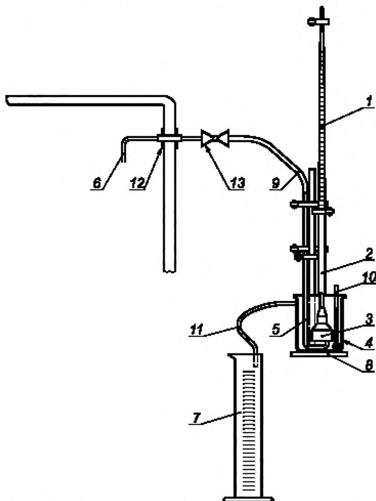
1 — бюретка 50 мл; 2 — резиновая трубка; 3 — воронка с цилиндрическим краем; 4 — емкость 2000 мл; 5 — трубка забора пара; 6 — капиллярная пробоборная трубка; 7 — измерительный цилиндр 250 мл; 8 — штатив бюретки; 9 — резиновая трубка; 10 — система измерения температуры; 11 — переливная трубка; 12 — ввод; 13 — управляющий клапан
