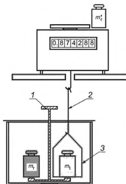
1 — устройство для смены гири; 2 — проволоочная подвеска; 3 — держатель для гири
