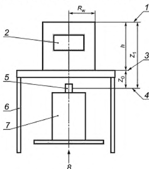
Рисунок В.1 — Оборудование для определения магнитной восприимчивости и намагничивания. Метод измерителя магнитной восприимчивости
