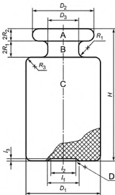
Рисунок B.8 — Иллюстрация определения объема цилиндрической гири (см. таблицу A.1)
