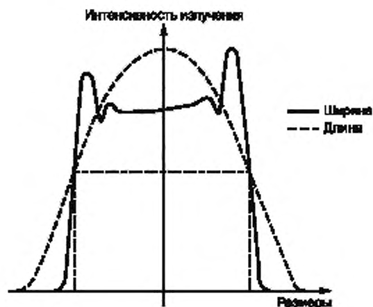
Рисунок С.2 — ФУНКЦИИ РАСШИРЕНИЯ ЛИНИИ для типичной РЕНТГЕНОВСКОЙ ТРУБКИ с большим ФОКУСНЫМ ПЯТНОМ (> 0,3 мм)
