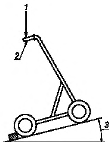
1 — нагрузка; 2 — задняя контрольная точка рукоятки; 3 — угол наклона
