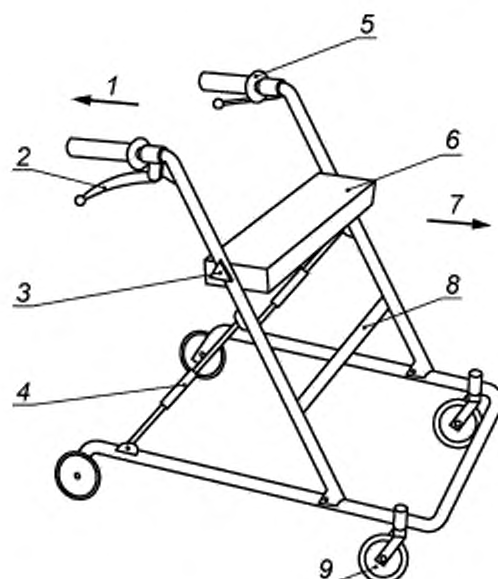
1 — направление назад; 2 — ручья тормоза; 3 — механизм регулирования высоты; 4 — механизм складывания; 5 — ручьятка/ручка; 6 — сиденье для отдыха; 7 — направление вперед; 8 — растяжка; 9 — колесики
