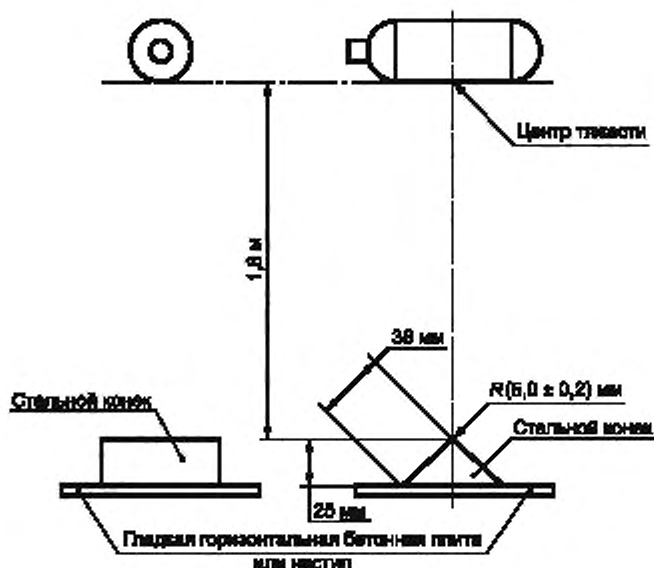
Рисунок 1 — Испытание контейнера падением на конек
