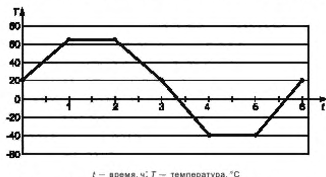
Рисунок 3 — Примерный цикл испытания на термостойкость
