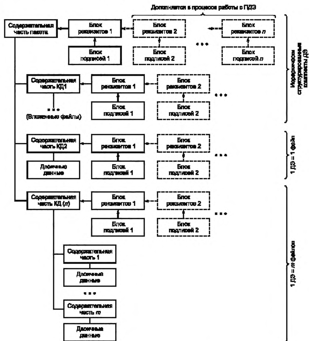
Рисунок В.1 — Логическая структура ПЭД
