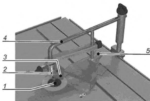
Рисунок М.304 — Направляющая
