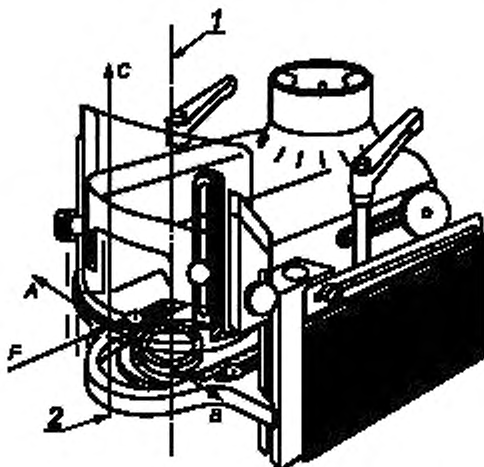
Рисунок М.310 — Определение точки измерения смещения регулируемого ограждения и направления приложения сил
