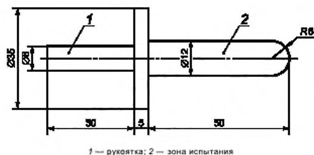
Рисунок М.306 — Испытательный щуп
