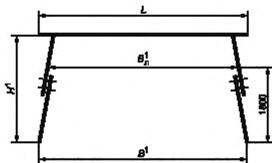
Рисунок 1 — Схема трапецевидной крепи (стойки могут быть криволинейными)
