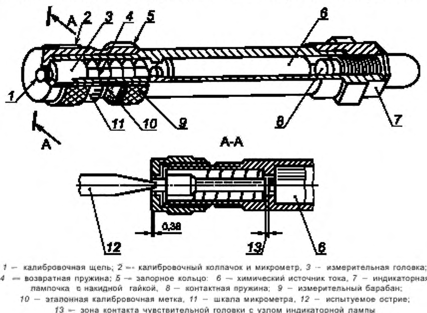
Рисунок 17 — Устройство для испытания концов
