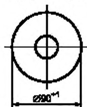
Рисунок 20 — Испытательный зонд С
