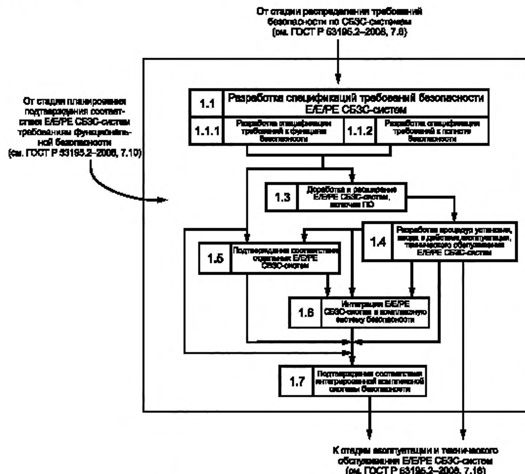
Рисунок 2 — Детализация стадии реализации жизненного цикла Е/Е/РЕ СБЗС-системы
