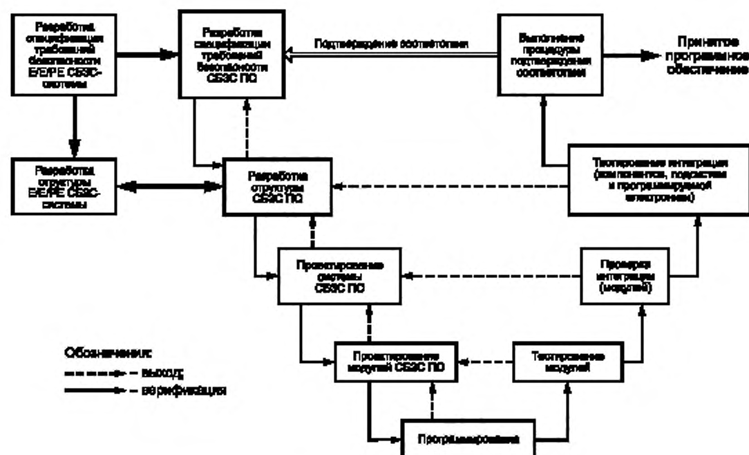
Рисунок 4 — V-модель проектирования и разработки СБЭС ПО
