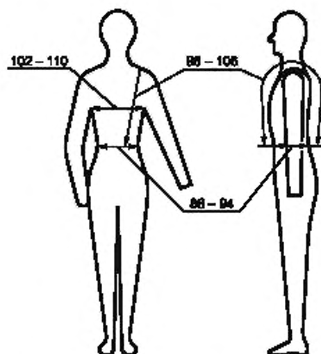
Рисунок D.2 — Средство защиты торса для мужчин
