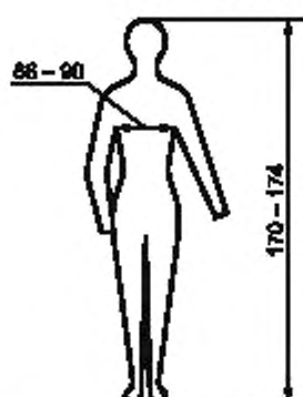
Рисунок D.2 — Минимальные требования к брюкам
