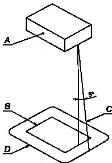
Рисунок 7 — Участок основания кожуха, который сконструирован в соответствии с 9.2.1, перечисления б) 1)
