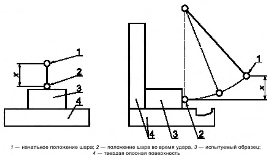
Рисунок 4 — Испытание на удар с помощью шара
