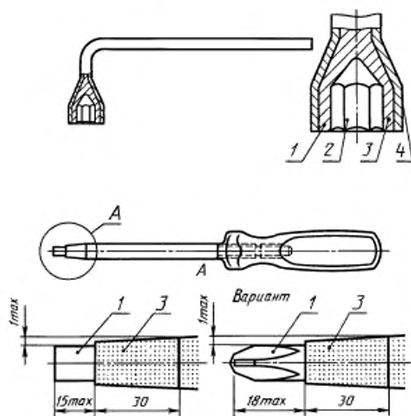
Рисунок 1 — Типы изоляции инструментов
