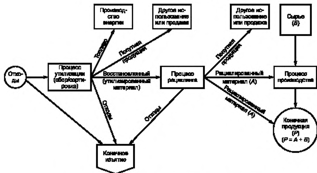
Рисунок А.1 — Упрощенная схема представления системы рециклинга
