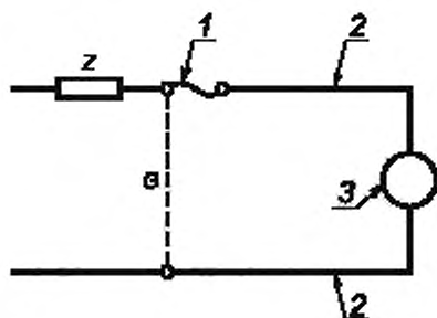
1 — предохранитель; 2 — испытуемый проводник; 3 — защитное устройство двигателя
