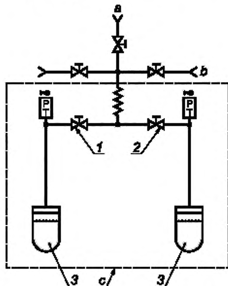
1 — вентиль раствора 1; 2 — вентиль раствора 2; 3 — испытуемый образец; а — воздушный клапан к вытяжному шкафу; б — источник газообразного азота; с — нагреваемое пространство
