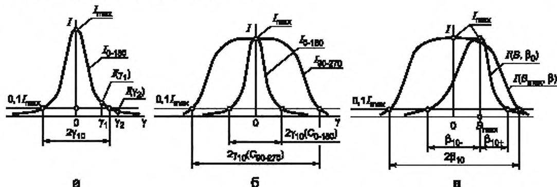
Рисунок 3 — Определение углов рассеяния прожектора
