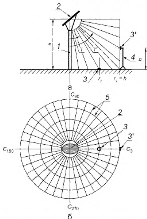
1 — стойка осветительного устройства, содержащая лампу (световод); 2 — отражающий экран; 3 и 3' — фотометрическая головка в положении измерения горизонтальной и вертикальной освещенности соответственно; 4 — раздвижной штатив; 5 — измерительная сетка горизонтальной плоскости в системе C , \gamma ;
