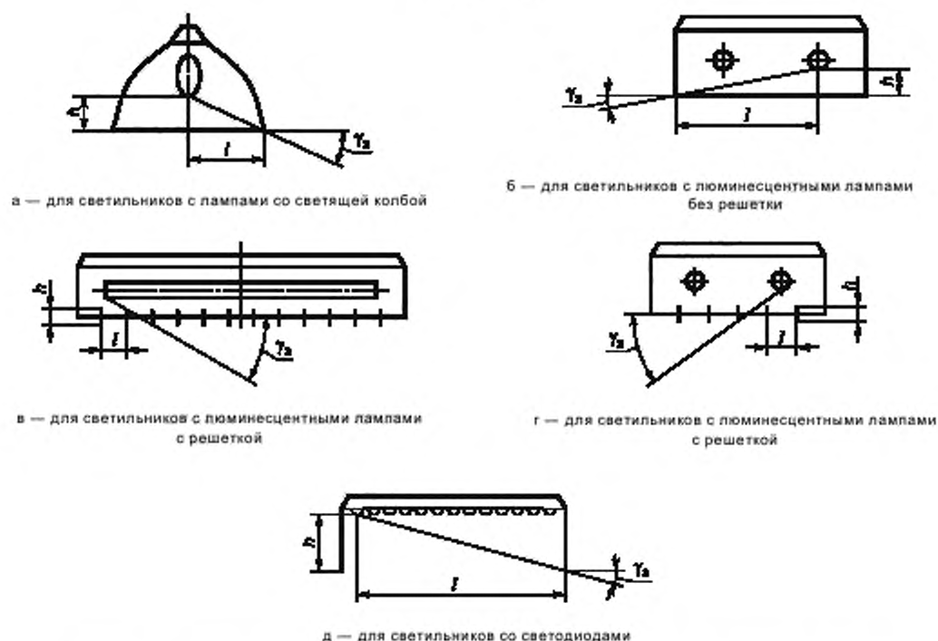
Рисунок 4 — Определение защитного угла светильника измерением конструктивных параметров
