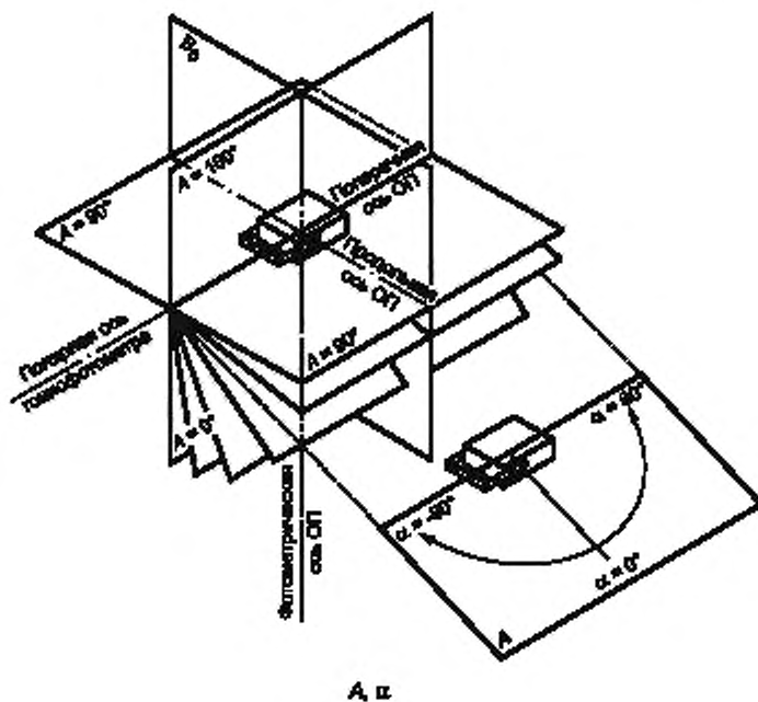
Рисунок Б.1, лист 2
