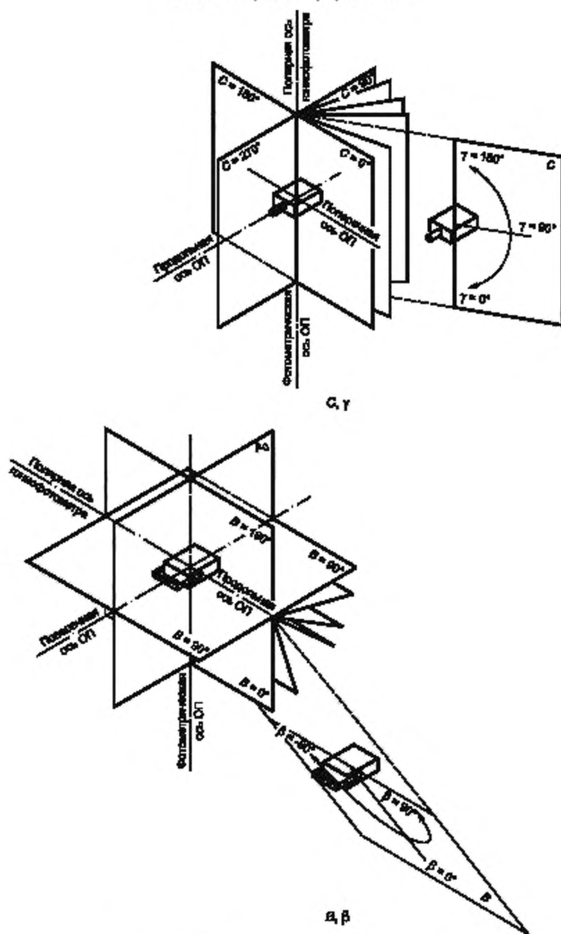
Рисунок Б.1 — Системы фотометрирования, лист 1
