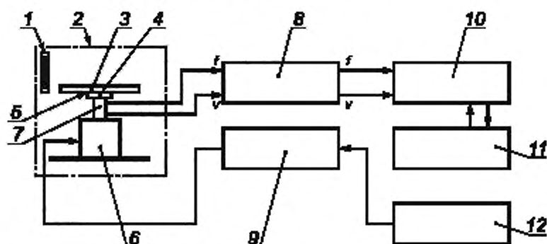
Испытательная установка
