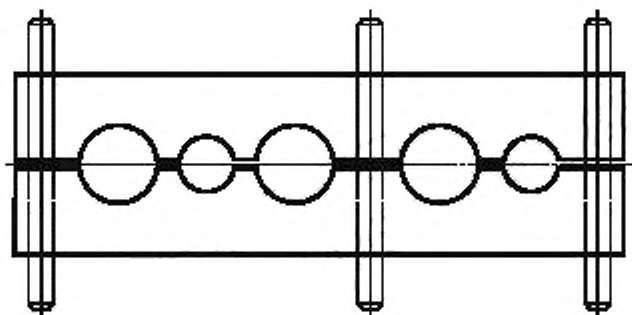
Рисунок 3 — Многоручьева колодка с промежуточным крепежным отверстием
