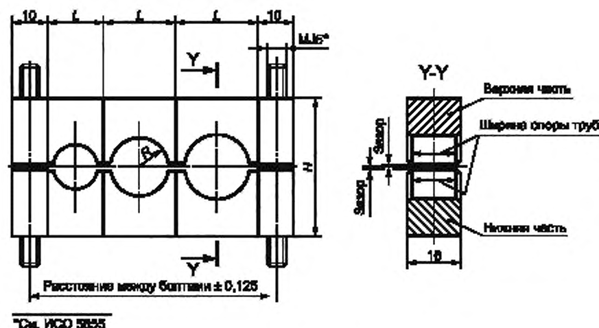
Рисунок 2 — Модульная колодка
