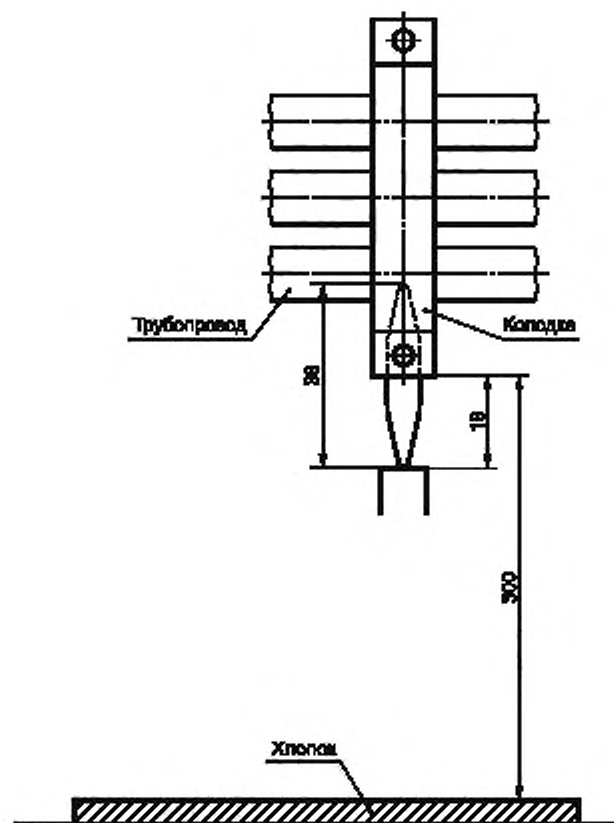
Рисунок 5 — Схема, показывающая положение колодки к пламени
