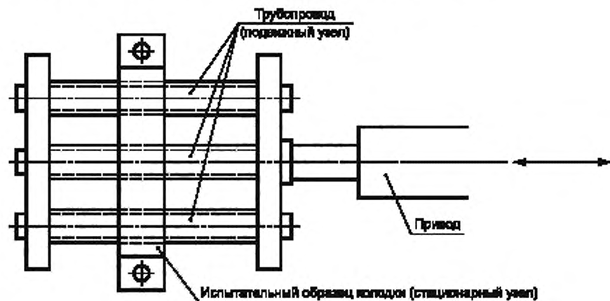
Рисунок 4 — Установка для испытаний на скольжение
