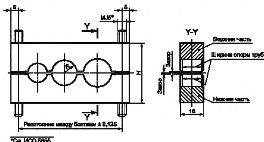
Рисунок 1 — Моноблочная колодка
