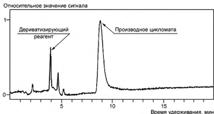
Рисунок В.2 — Хроматограмма земляничного йогурта
