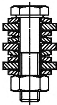
Рисунок 4 — Испытательное приспособление для тарельчатых пружинных шайб
