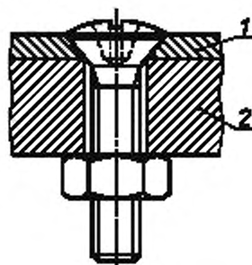
1 — верхняя пластина с зенковкой; 2 — нижняя пластина
