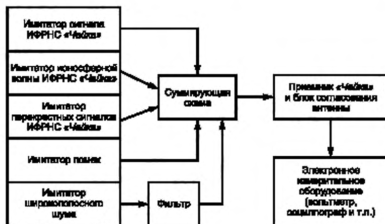
Рисунок 1 — Типовое испытательное оборудование
