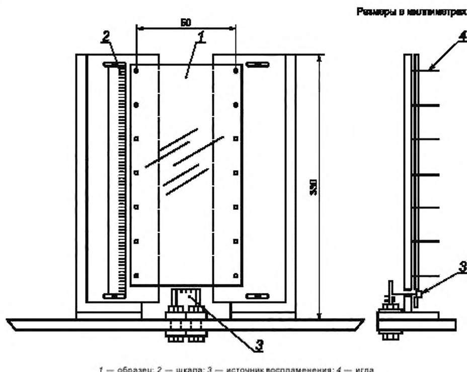
Рисунок 2 — Держатель с игольной поверхностью для тонкослойных образцов
