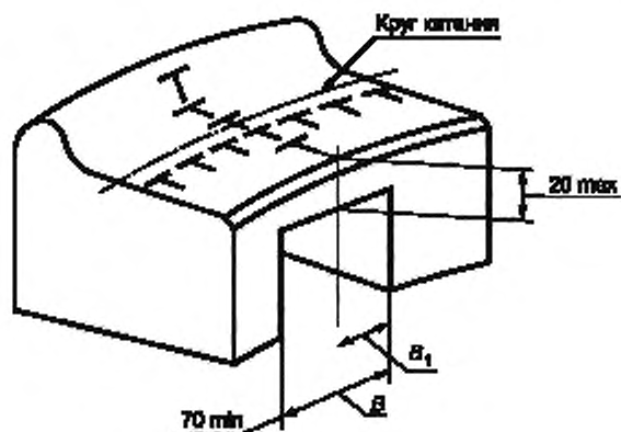
Рисунок А.4 — Схема установки тензорезисторов на бандаже или ободе колеса и механическое поднутрение фрагмента бандаж в поперечном направлении
