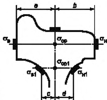
Рисунок А.6 — Схема приведения к плоскости круга катания ( \sigma_{ср} и \sigma_{ср1} ) напряжений замеренных ( \sigma_B , \sigma_H , \sigma_{B1} , \sigma_{H1} ) на боковых поверхностях обода (бандаж) и приободной части диска
