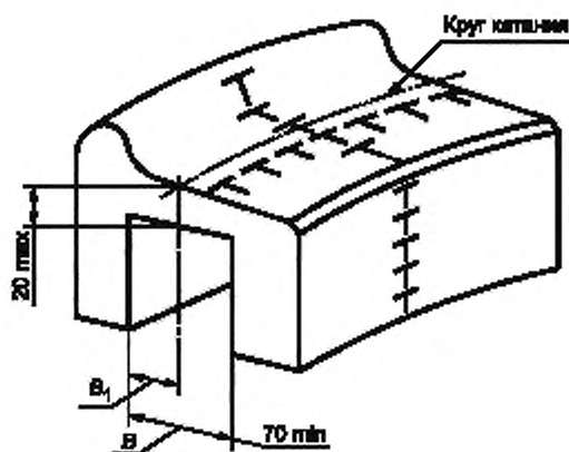
Рисунок А.4 — Схема установки тензорезисторов на бандаже или ободе колеса и механическое поднутрение фрагмента бандаж в поперечном направлении
