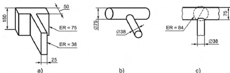
Рисунок 5 — Модели эквивалентного круга. Труба (любого сечения)
