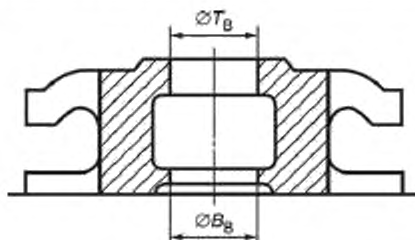
Рисунок 10 — Отверстия элеваторов для обсадных и насосно-компрессорных труб
