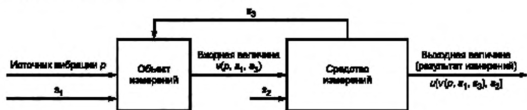
Рисунок 4 — Потенциальные источники помех
