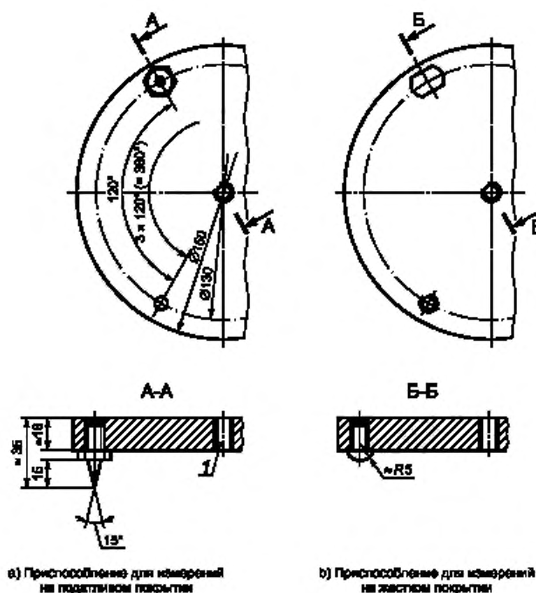
Рисунок 1 — Приспособления для быстрой установки датчиков вибрации
