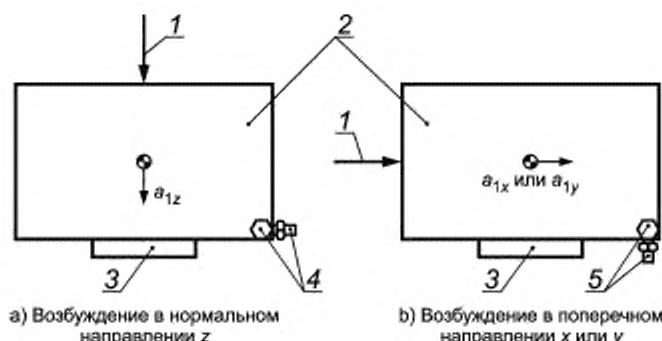
1 — вибровозбудитель; 2 — плита распределения вынуждающей силы; 3 — входной фланец испытуемого объекта; 4 — нежелательная вибрация a'_{1z} и a'_{1y} ; 5 — нежелательная вибрация a'_{1z} и a'_{1y} или a'_{1x}
