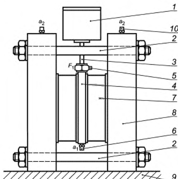
1 — вибровозбудитель; 2 — устройство предварительного статического нагружения; 3 — толкатель; 4 — плита распределения вынуждающей силы; 5 — датчик силы (измерение F_1 ); 6 — акселерометр (измерение a_1 ); 7 — номинально идентичные упругие опоры; 8 — жесткие вертикальные стойки; 9 — жесткий фундамент; 10 — акселерометр (измерение a_2 )
