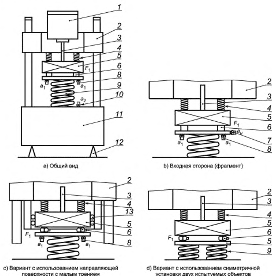
1 — вибровозбудитель; 2 — траверса; 3 — толкатель; 4 — вспомогательные виброизоляторы (статическая нагрузка); 5 — плита распределения вынуждающей силы; 6 — датчик силы (измерение F_1 ); 7 — акселерометр (измерение ускорения a_u в направлении нежелательного возбуждения); 8 — акселерометр (измерение a_1 ); 9 — испытуемый объект; 10 — акселерометр (измерение a_2 ); 11 — жесткий фундамент; 12 — подвеска; 13 — направляющая поверхность с малым трением
