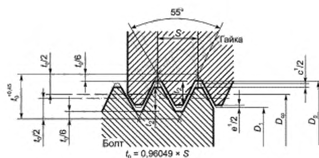
Рисунок Б.1 — Внутренняя резьба резьбового кольца
