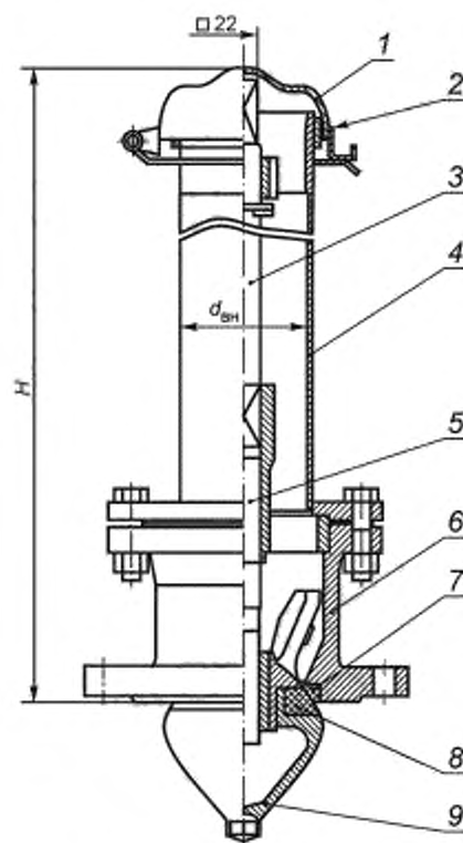
1 — крышка; 2 — nipple; 3 — штанга; 4 — корпус; 5 — шпилька; 6 — патрубок; 7 — седло; 8 — кольцо уплотнительное; 9 — клапан
