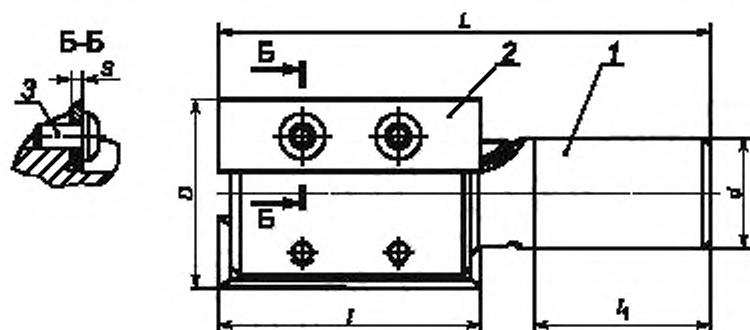
1 — корпус; 2 — пластина или нож; 3 — крепежный элемент
