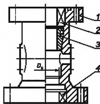
1 — корпус; 2 — верхний уплотнитель; 3 — трубодержатель; 4 — нижний уплотнитель
