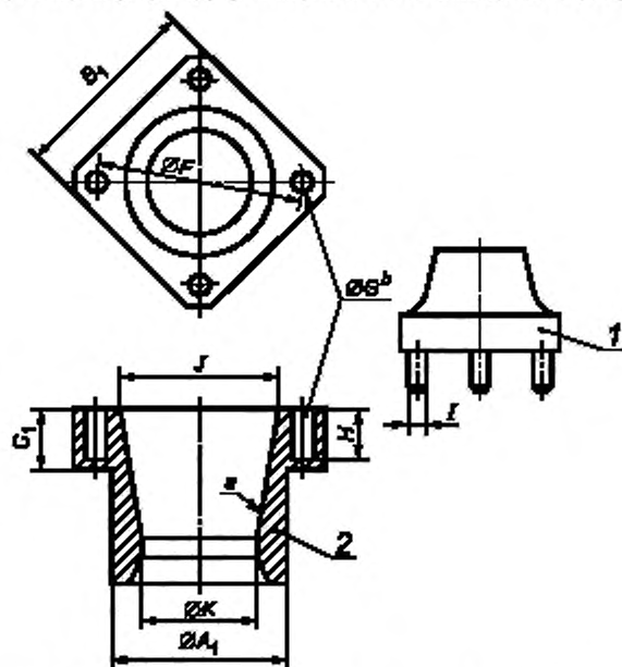
1 — вкладыш ротора под ведущую трубу с ведущими пальцами. 2 — постоянная втулка. a — конусность 1:3 (330 ± 1,5) мм/м, b — диаметр поводкового отверстия
