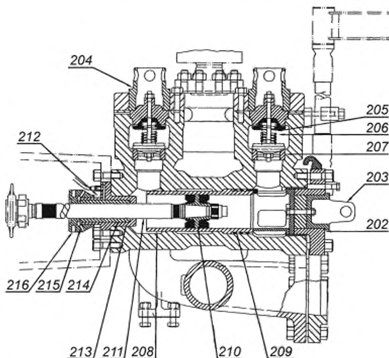
Рисунок В.4 — Нагнетательная часть duplexного бурового насоса двукратного действия (номенклатуру деталей см. в таблице В.2)
