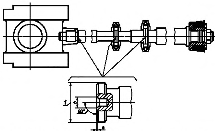
1 — диаметр торца; а — плоские поверхности контакта и посадочные диаметры на сопряженных соединениях удлинения ползуна со ступицей поршня в буровых насосах; б — допуск осности между осевой линией посадочного диаметра и теоретической осью штока не должен превышать 0,13 мм
