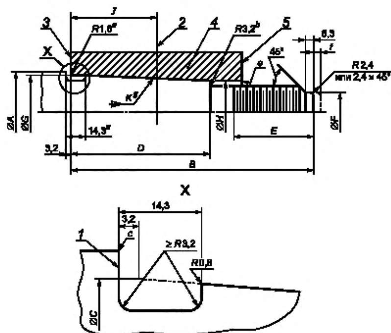
1 — запящик штока М, 2 — геометрическая ось поршня (в сборе) 3 — запящик N, запящик поршня, штоковая полость: а — максимальный размер; б — минимальный размер; с — фаска \leq 0,5 мм; J — длина до центральной оси поршня, В — длина штоковой полости; X — галтель и диаметр выточки, нагнатованной при холодной обработке 4 — поршень, 5 — запящик Р, запящик поршня, конец резьбы: е — фаска, f — максимальное удлинение хвостовика 3,2 мм; g — конус; R — радиус или фаска
