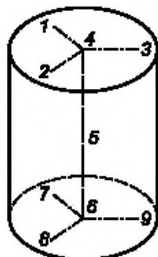
Рисунок Б.1 — Положение термопар (1 — 9) в цилиндрических печах
