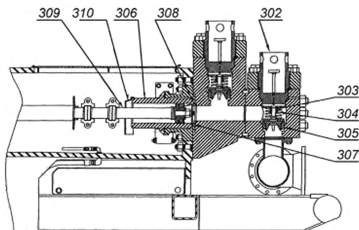
Рисунок В.5 — Нагнетательная часть триплексного бурового насоса одностороннего действия (номенклатура деталей см. в таблице В.3)
