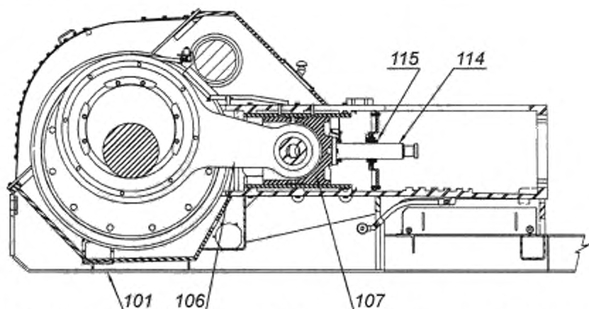
Рисунок В.1 — Поперечное сечение нагнетательной части (номенклатура деталей см. в таблице В.1)
