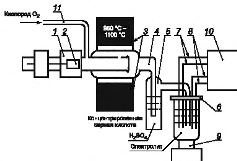
1 — приемник образца; 2 — кварцевая лодочка; 3 — печь для сжигания; 4 — кварцевая трубка для сжигания; 5 — абсорбер с концентрированной серной кислотой; 6 — титровальная ячейка с электролитом; 7 — рабочие электроды; 8 — измерительные электроды; 9 — электромагнитная мешалка; 10 — регистрирующее устройство для регистрации массовой концентрации галогенов; 11 — трубка для ввода кислорода для сжигания пробы
