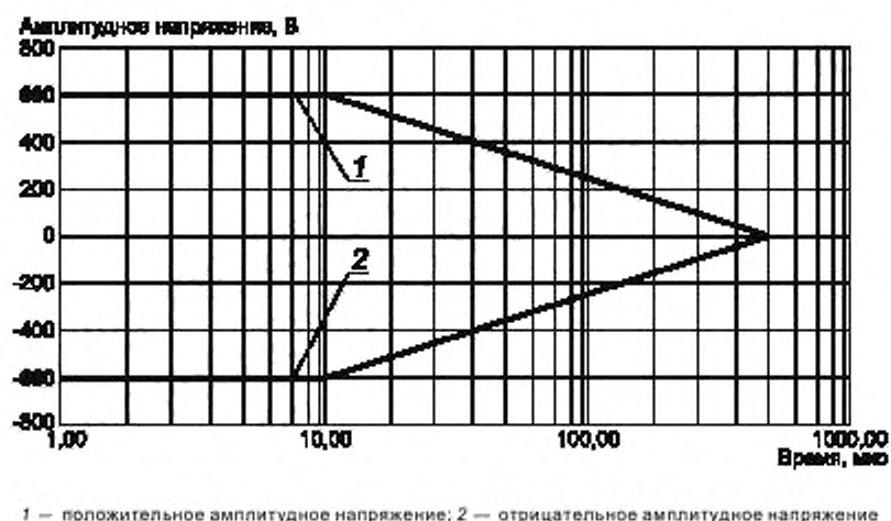
Рисунок 18 — Огибающая импульсов напряжения для приемников постоянного и переменного токов
