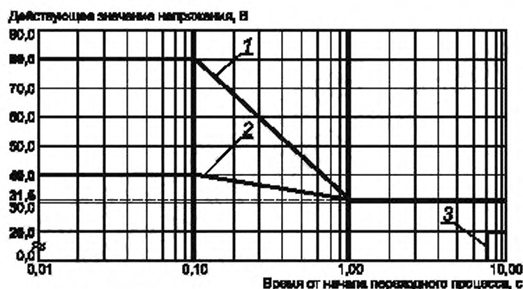
Рисунок 11 — Пределы ненормальных повышенных и пониженных напряжений первичных систем постоянного тока 27 В
