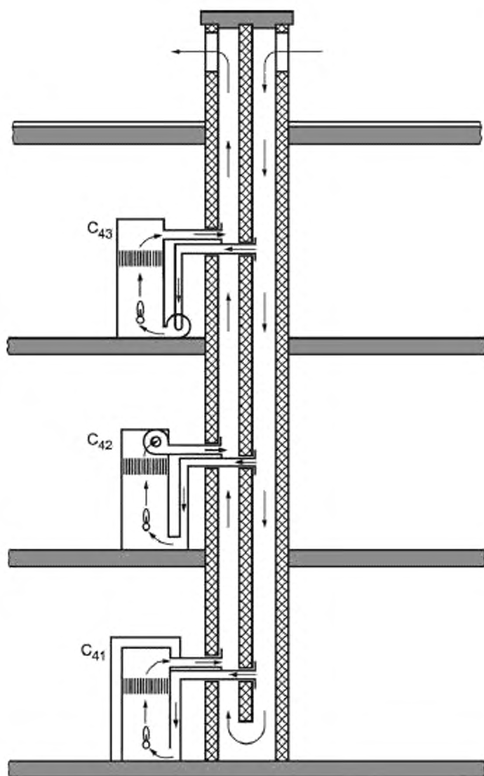
Рисунок В.4 — Водонагреватели типа C_4
