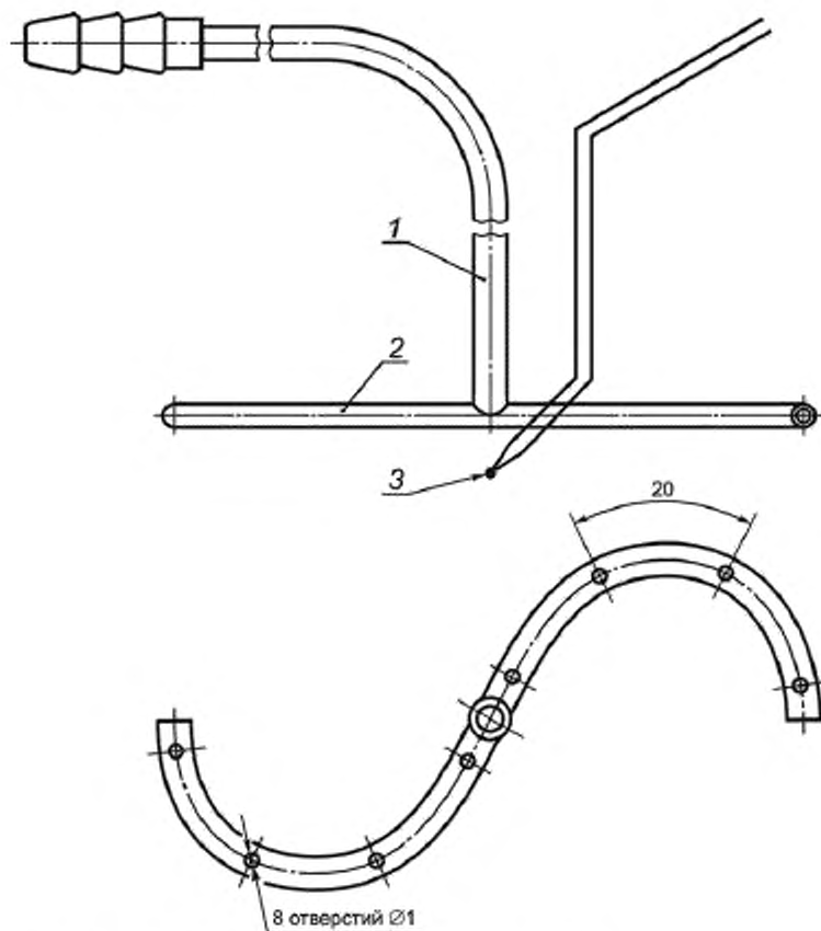
1 — медная трубка \varnothing 6 мм; 2 — медная трубка \varnothing 4,3 мм; 3 — термопара
