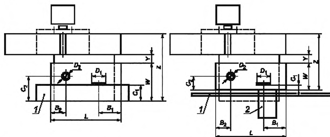
1 — встроенный передвижной стол; 2 — дополнительный передвижной стол (каретка); B_1 — расстояние между осью шпинделя дисковой пилы и передней боковой кромкой встроенного передвижного пильного/фрезерного стола; B_2 — расстояние между осью фрезерного шпинделя и задней боковой кромкой встроенного передвижного пильного/фрезерного стола; C_1 — расстояние между полотном дисковой пилы и кромкой дополнительного передвижного пильного/фрезерного стола (каретки); C_2 — расстояние между осью фрезерного шпинделя и передней кромкой встроенного передвижного пильного/фрезерного стола; D_1 — диаметр основной фрезы, D_2 — диаметр отверстия в столе; L — длина дополнительного передвижного пильного/фрезерного стола (каретки); Y — ширина зазора между пильным/фрезерным и фуговальным столами; Z — расстояние между передней кромкой фуговального стола и передней кромкой дополнительного передвижного пильного/фрезерного стола (каретки); W — расстояние между передним краем передвижного пильного/фрезерного стола и передним краем каретки.
