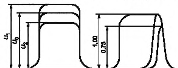
Рисунок 5 — Примеры выходного сигнала на экране осциллографа
