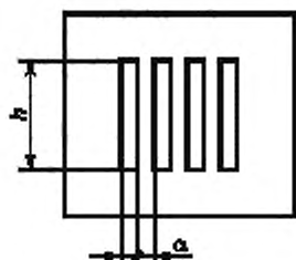
Рисунок В.1 — Набор четырехштриховых миш для измерения минимальной разрешаемой разности температур
