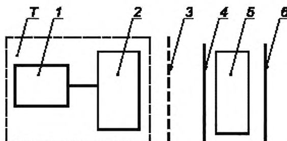
Т — испытуемый тепловизор (1 — блок регистрации, 2 — оптическая головка); 3 — нейтральный ослабляющий фильтр; 4 — штриховая мира; 5 — излучатель-термостат; 6 — экран-фон
