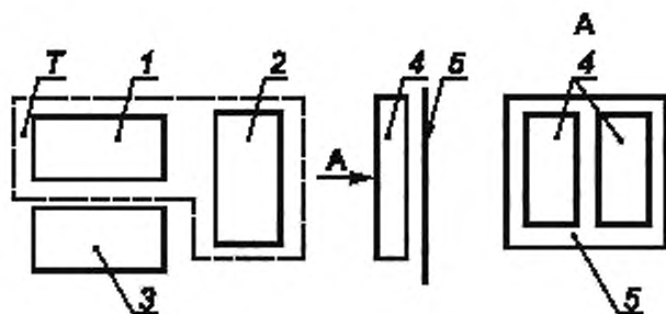
Т — испытуемый тепловизор (1 — блок регистрации; 2 — оптическая головка); 3 — прибор для регистрации термопрофиля, 4 — излучатели-термостаты; 5 — экран-фон
