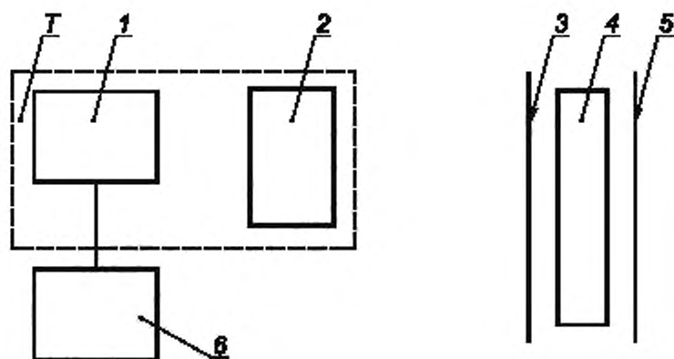
Т — испытуемый тепловизор (1 — блок регистрации, 2 — оптическая головка); 3 — щелевая мишень; 4 — излучатель-термостат; 5 — экран-фон, 6 — осциллограф
