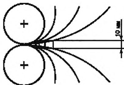
Рисунок 12 — Измерение безопасного расстояния в местах затягивания
