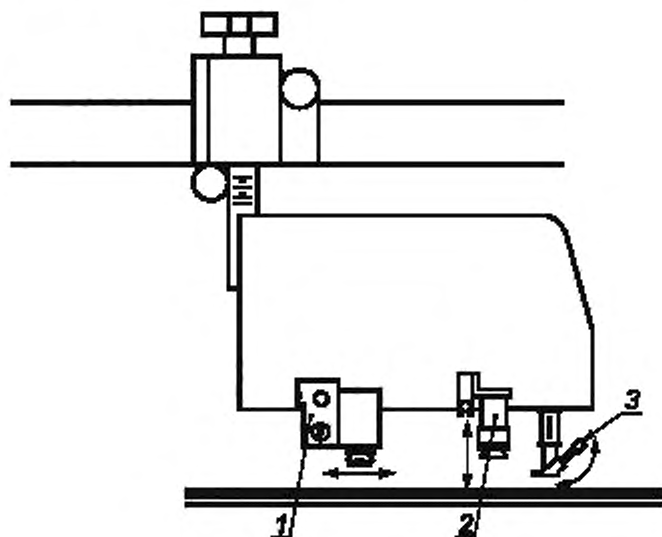
1 — листоведущий присос; 2 — листоотделяющий присос; 3 — шуп-сопло («сапожок»)
