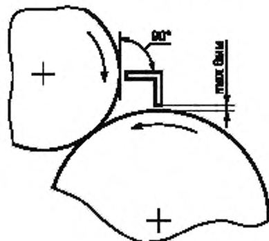
Рисунок 3 — Защита места затягивания с помощью неподвижной планки
