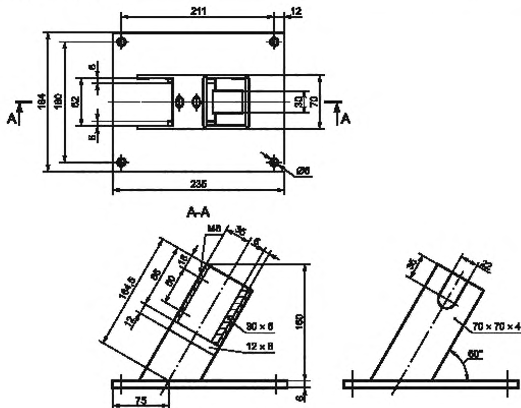
Рисунок 8 — Опорный стенд
