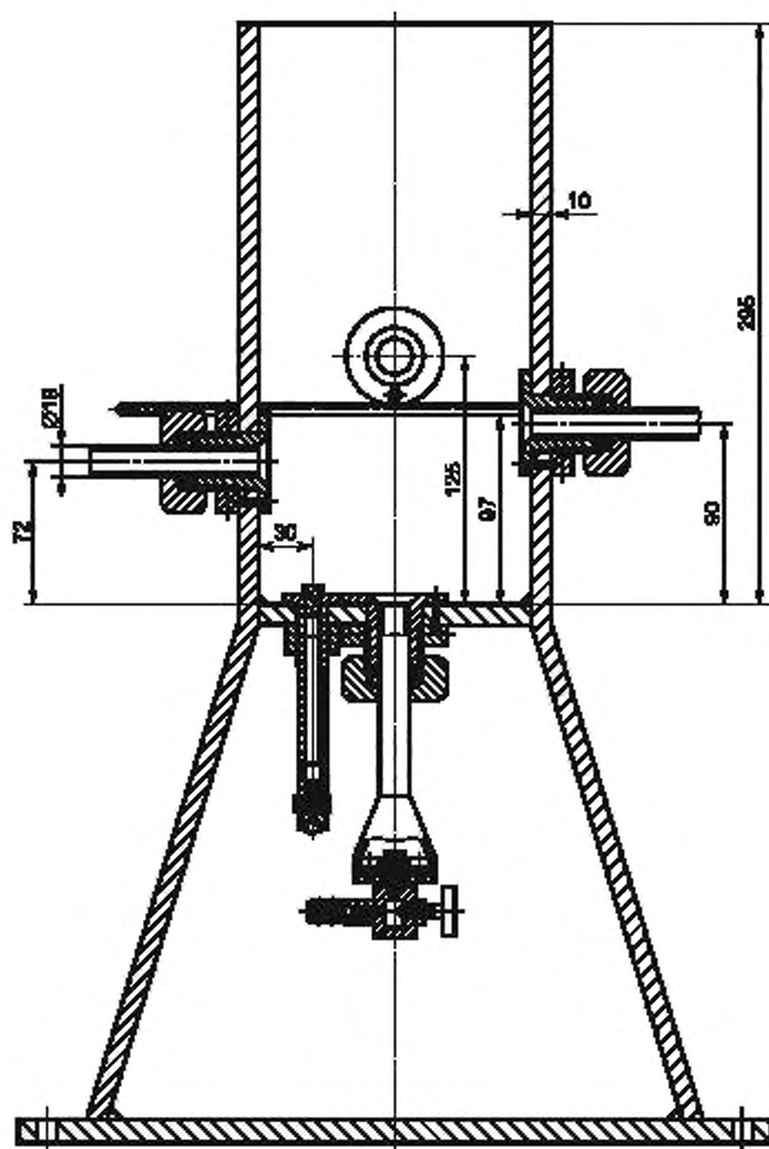
Рисунок 5 — Защитно-нагревательное устройство
