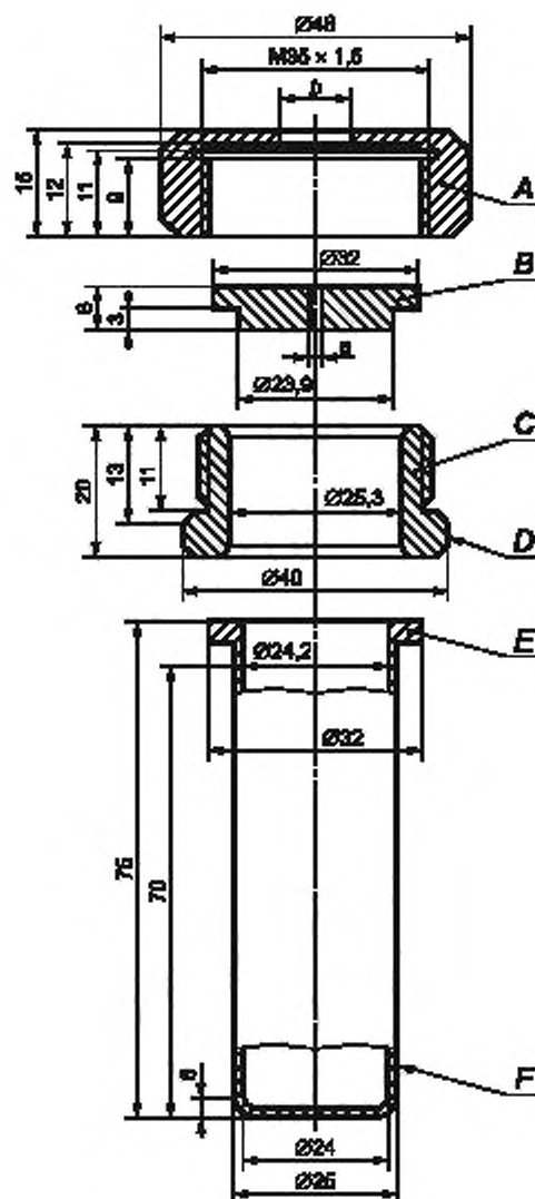
Рисунок 4 — Прибор для проведения испытания по Кюену (опытный комплект с трубкой)
