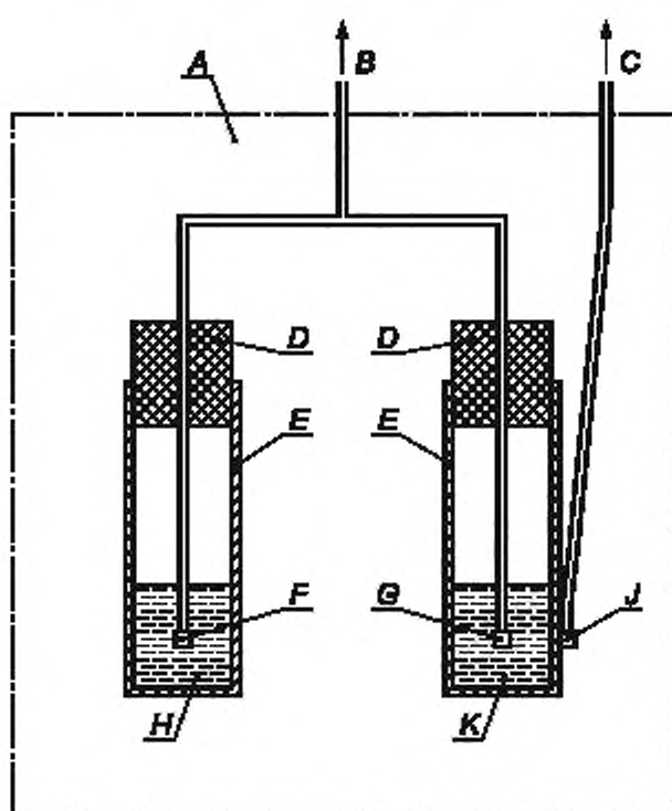
A — печь; B — к милливольтметру ( T_1 - T_2 ); C — к милливольтметру ( T_3 ); D — пробки; E — пробирки; F — термодатчик № 1 ( T_1 ); G — термодатчик № 2 ( T_2 ); H — 100\text{ см}^3 образца; J — термодатчик № 3 ( T_3 ); K — 100\text{ см}^3 эталонной химической продукции
