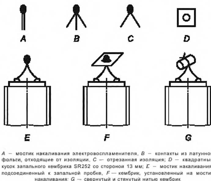
Рисунок 9 — Система зажигания для твердой химической продукции
