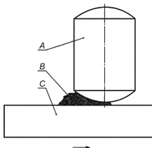
А — фарфоровый шпindel, 10 × 15 мм, В — опытный образец; С — фарфоровая пластина 25 × 25 × 15 мм
