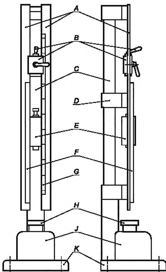
А — две направляющие рейки; В — захватно-пусковое устройство; С — стойка; D — средняя перекладина; E — падающий груз; F — зубчатая рейка; G — градуированная шкала; H — наковальня (100 мм (диам.) × 70 мм); J — стальной блок, 230 × 250 × 200 мм; K — основание, 450 × 450 × 60 мм
