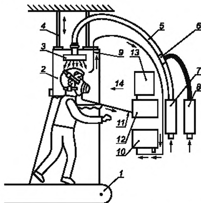
1 — беговая дорожка; 2 — камера; 3 — распределитель потока; 4 — подвеска; 5 — шланг подачи тест-вещества; 6 — место разбавления SF_6 воздухом; 7 — расходомер воздуха, оснащенный контрольным устройством; 8 — расходомер SF_6 , оснащенный контрольным устройством; 9 — пробоотборник для отбора тест-вещества; 10 — прибор для измерения концентрации тест-вещества; 11 — трубка отбора проб для определения концентрации тест-вещества; 12 — прибор для измерения концентрации тест-вещества во вдыхаемом воздухе; 13 — регистрирующее устройство; 14 — воздух для дыхания, не содержащий тест-вещество
