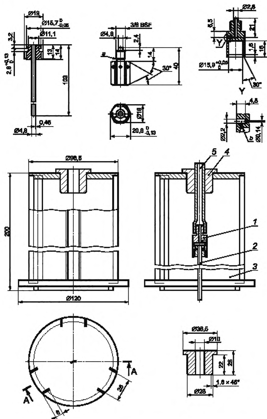
1 — солло; 2 — подающая труба (раствор соли); 3 — рукав (изготовленный из непластифицированного ПВХ); 4 — втулка; 5 — трубка для воздуха (диаметр — 10,0 мм)
