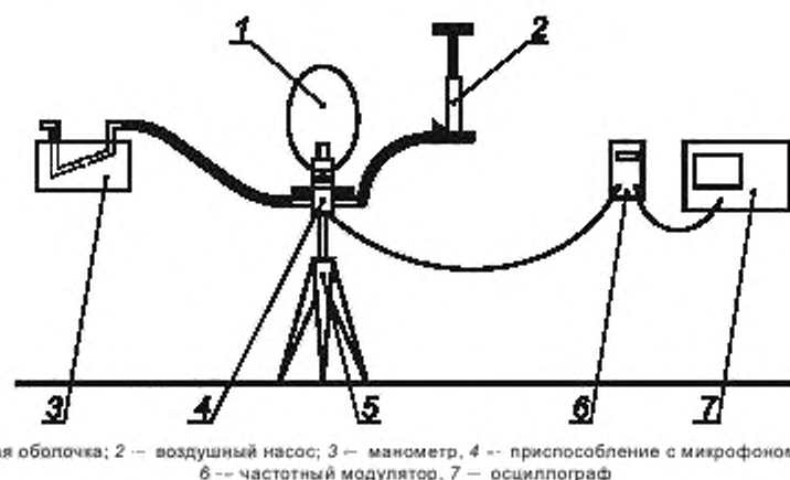
Рисунок В.2 — Пример установки для калибровки микрофона
