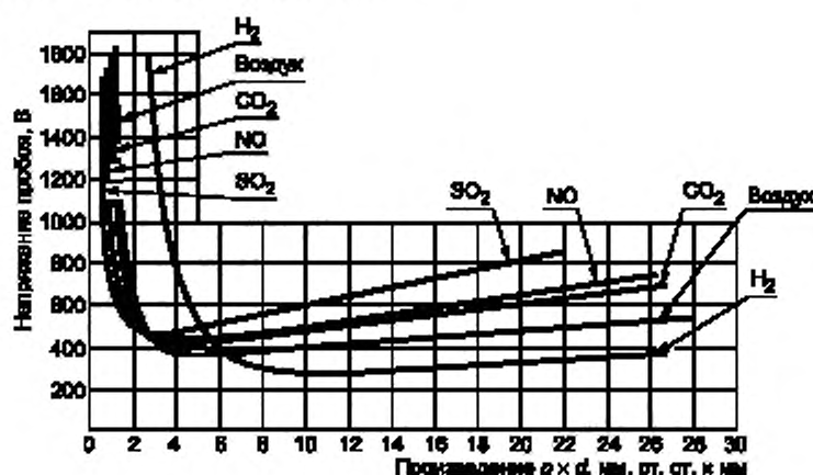
Рисунок 1 — Кривая Пашена
