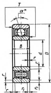
Типы 36000, 36000K6, 46000, 66000
