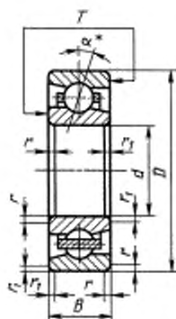
Тип 26000K
