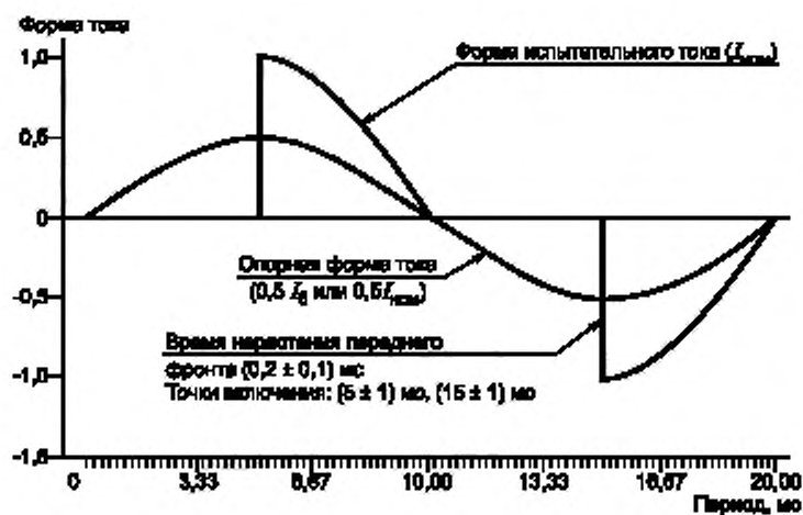
Рисунок A.5 — Форма тока при фазовом управлении
