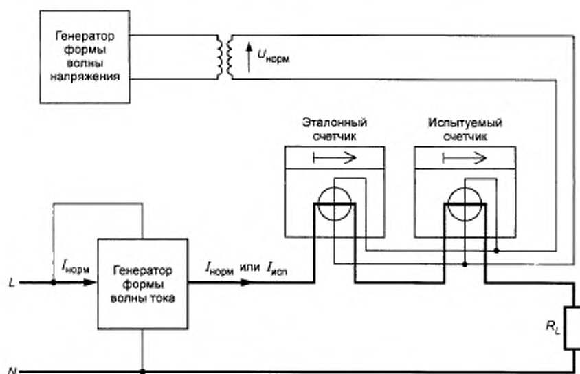
Рисунок A.4 — Схема испытательной цепи (справочная)
