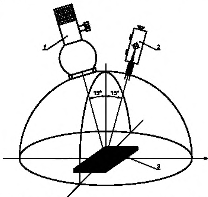
Рисунок 40 — Конфигурация для оценки коэффициента яркости \beta
