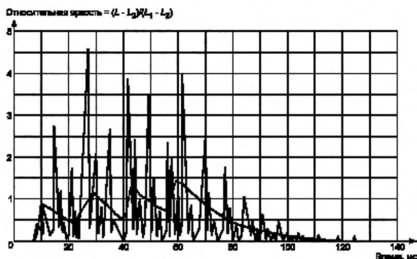
Рисунок 42 — Пример характеристики яркости до и после фильтрации. Время формирования изображения 71 мс
