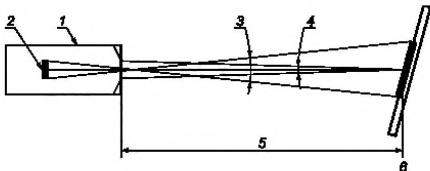
1 — фотометр; 2 — фоточувствительный элемент; 3 — поле обзора = поле зрения = угловой размер рассматриваемого объекта; 4 — приемный конус. Угол, образованный входным лучом прибора на рабочем расстоянии; 5 — рабочее расстояние. Расстояние между передней линзой прибора и рассматриваемым объектом, который прибор может сфокусировать; 6 — EUT = испытуемое оборудование (см. 3.1.4)
