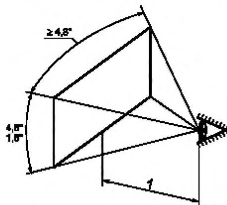
Рисунок 10 — Панель малых размеров
