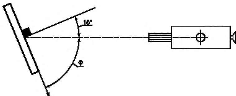
Рисунок 39 — Геометрия измерения для оценки отражения
